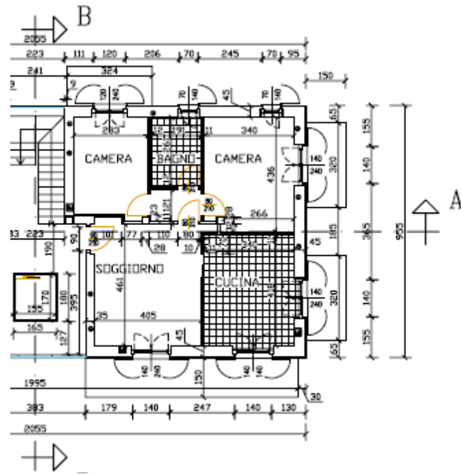
TRILOCALE AL PIANO PRIMO
